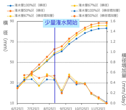
図3 初秋の少量かん水が「甘平」果実肥大に及ぼす影響
