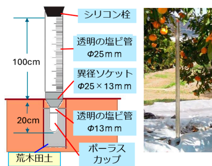
図1 簡易土壌水分計の概要と設置状況（原図：西日本農研センター）
