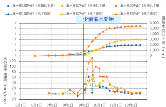
図2 簡易土壌水分計の累積水位低下量と低下速度
