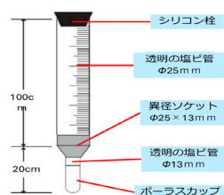
図2 簡易土壌水分計の概要と設置状況 (原図：西日本農研センター)
