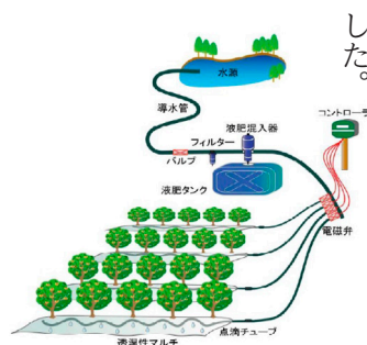
図1 マルドリ方式の概要 (原図 西日本農研センター)
