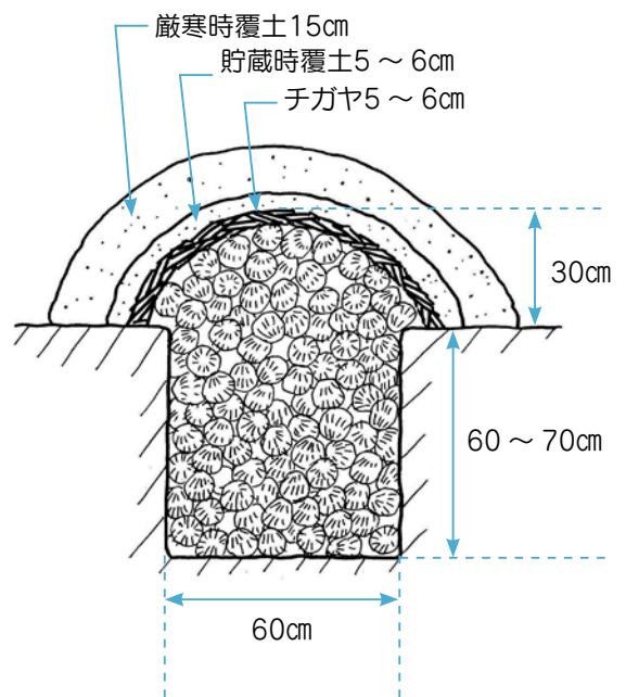
図3 サトイモの種芋貯蔵方法
